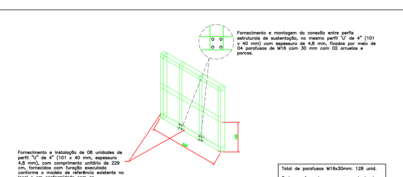
DETALHE 05 - SUBSTITUIÇÃO DA LONGARINA TRAVAMENTO LATERAL INFERIOR
