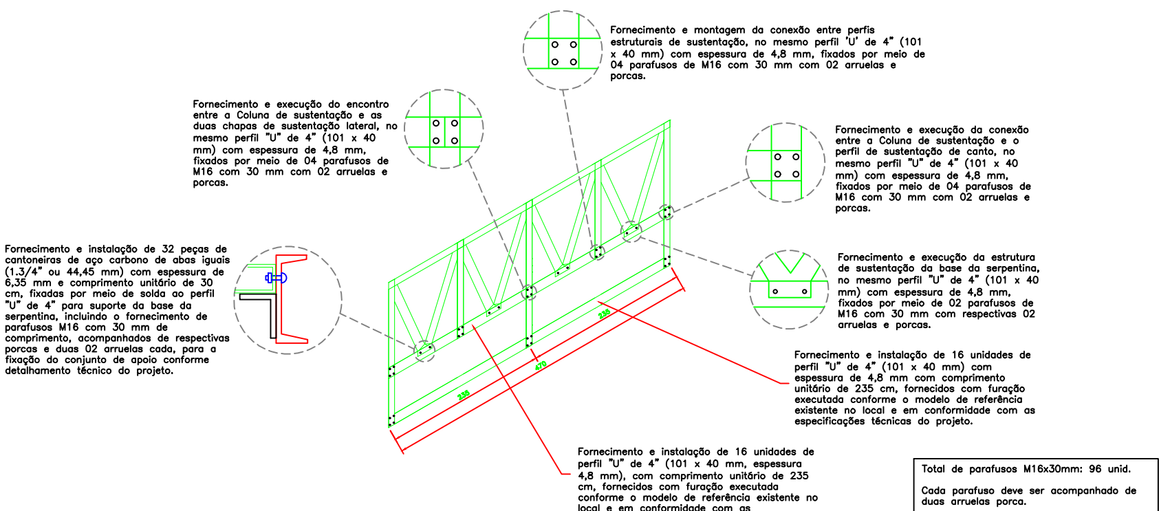
DETALHE 04 - SUBSTITUIÇÃO DA LONGARINA DE SUSTENTAÇÃO DAS SERPENTINAS E TRAVAMENTO FRONTAL MEIO E INFERIOR
