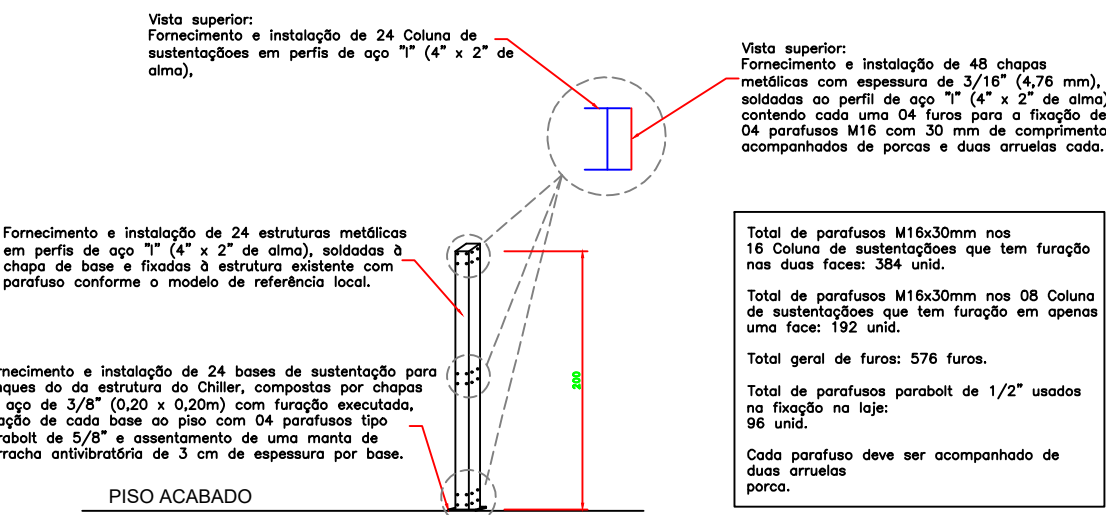
DETALHE 01 - NOVO SUPORTE DE SUSTENTAÇÃO DO MÓDULO DO CHILLER
