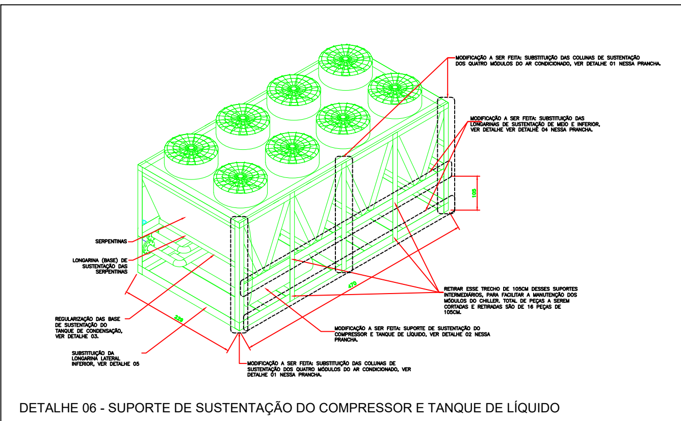
DETALHE 06 - SUPORTE DE SUSTENTAÇÃO DO COMPRESSOR E TANQUE DE LÍQUIDO
